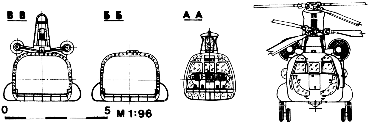
CH-47D
