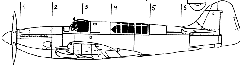
"Файрфлай" Mk. V
