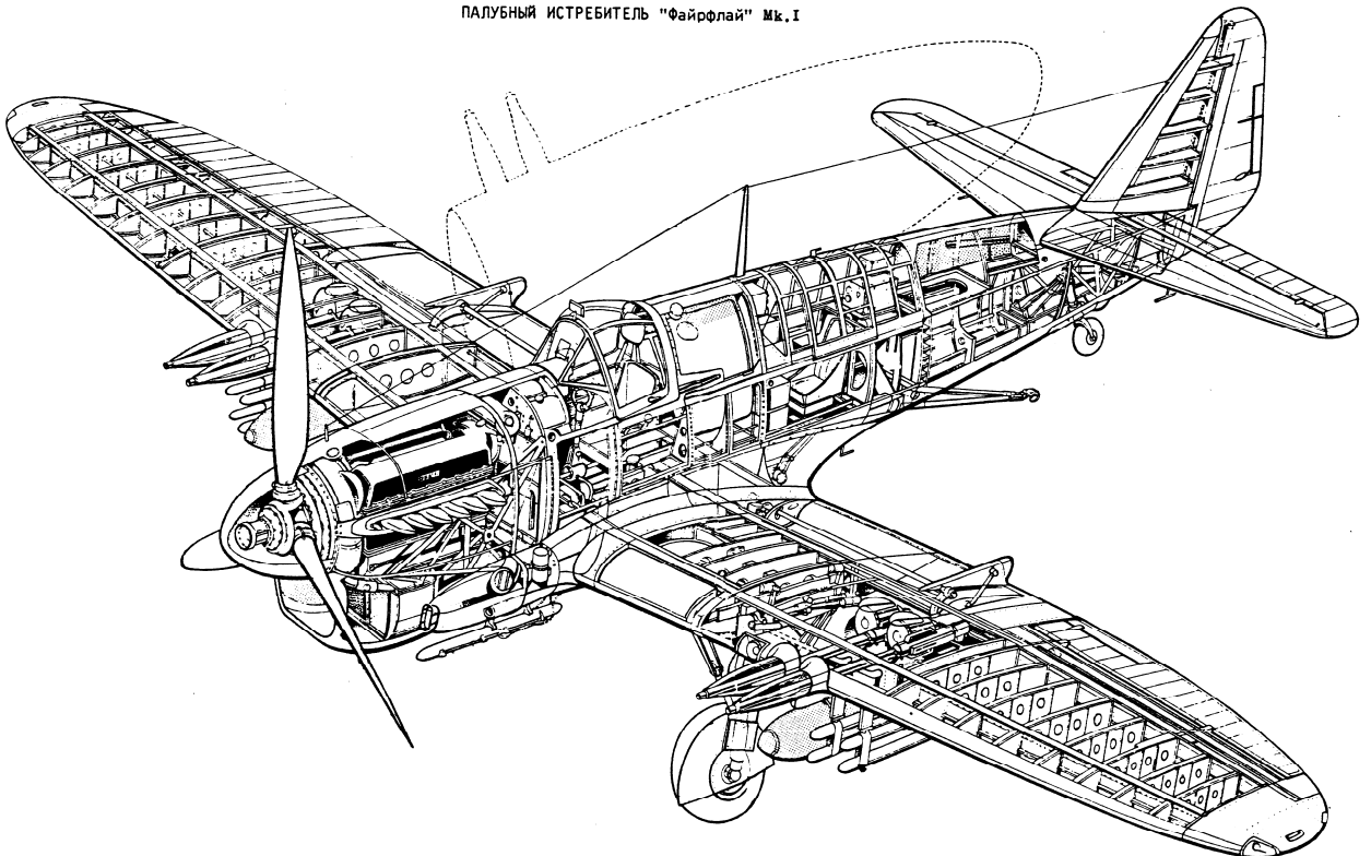
ПАЛУБНЫЙ ИСТРЕБИТЕЛЬ "Файрфлай" Mk. I
