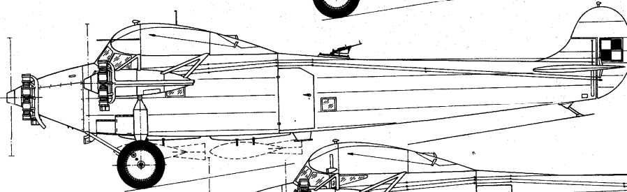
Чехословацкий "Авиа" F.VII B/3m
