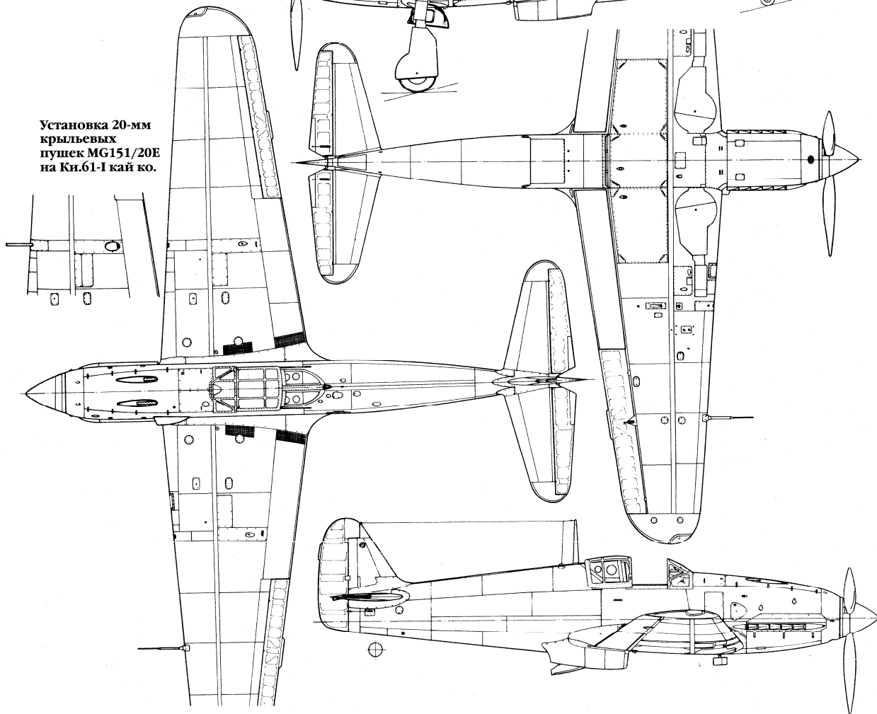
Ки.61-I оцу (левый борт, вид сверху, вид снизу, правый борт).
