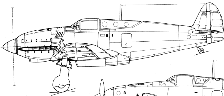
Первый прототип лёгкого (фронтового) истребителя Ки.6101 в полётной конфигурации (левый борт).
