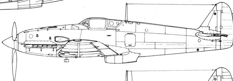
Первый прототип лёгкого (фронтового) истребителя Ки.6101 в полётной конфигурации (левый борт).
