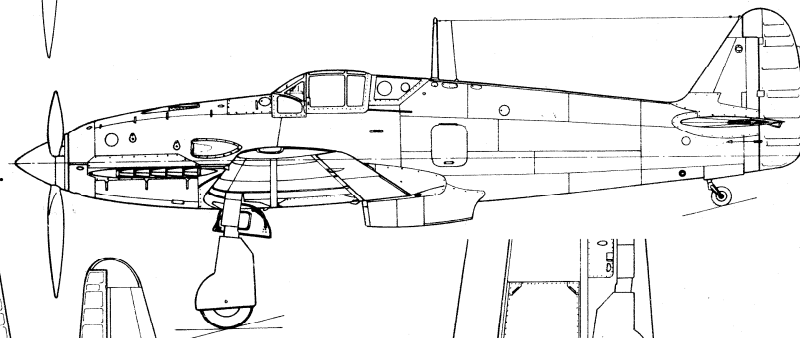
Ки.61-I оцу (левый борт, вид сверху, вид снизу, правый борт).
