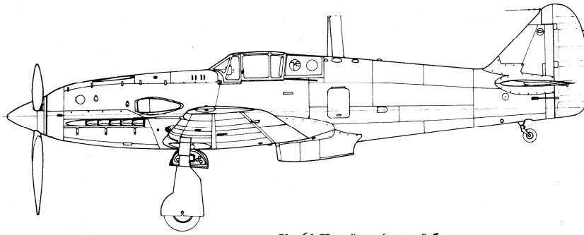
Ки.61-II кай ко (левый борт, вид снизу и вид сверху).
