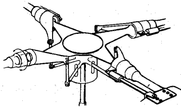
Втулка несущего ротора
