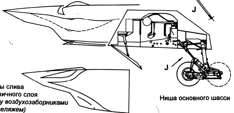
Разрез воздухозаборника (пунктиром указаны крайние положения регулируемого клина и нижней створки)
