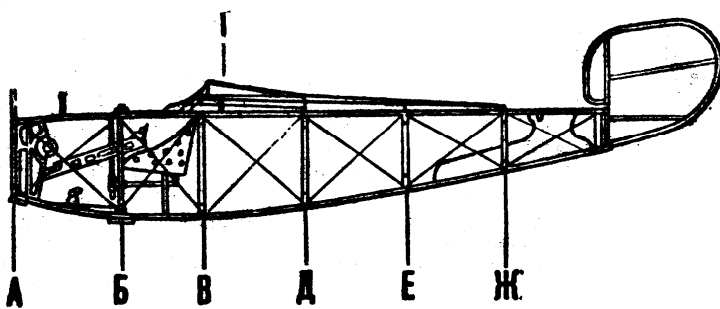
КАРКАС ФЮЗЕЛЯЖА
