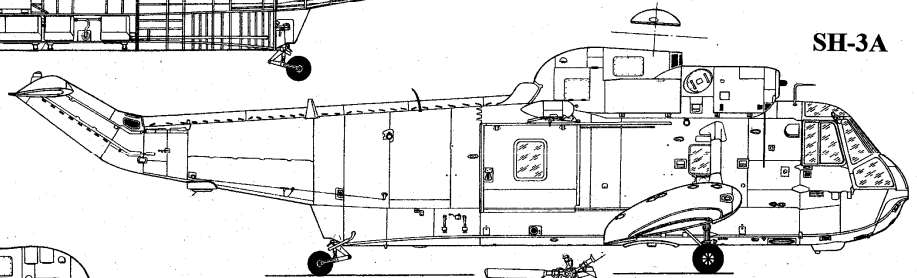
SH-3A продольный разрез
