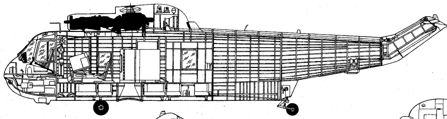
SH-3A продольный разрез
