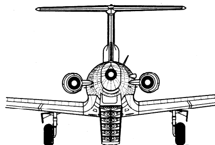
Як-40 (опытный образец)
