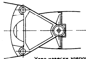
Узел навески элерона
