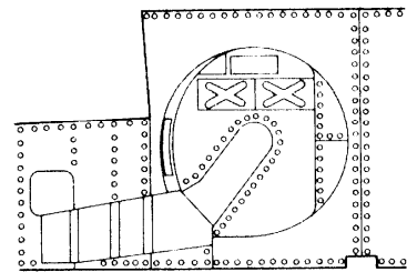
Ниша уборки шасси
